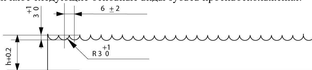
Рисунок 1.1 – S4 «Зубья пилы»
