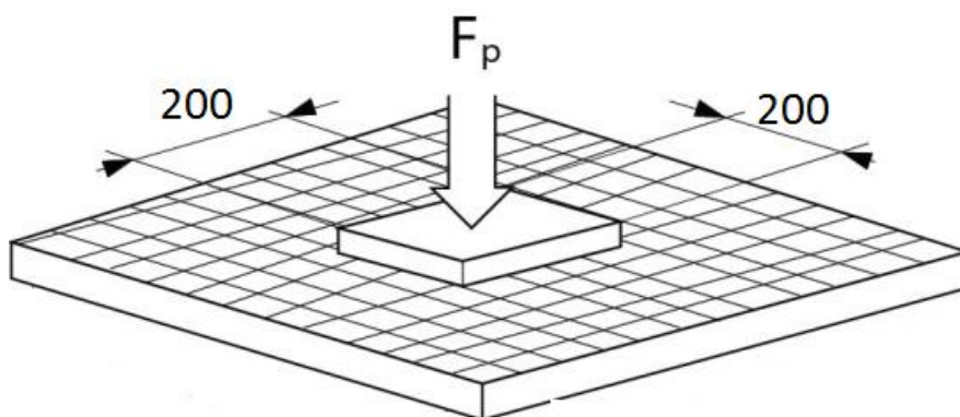
Рис.3.2. Сосредоточенная нагрузка
