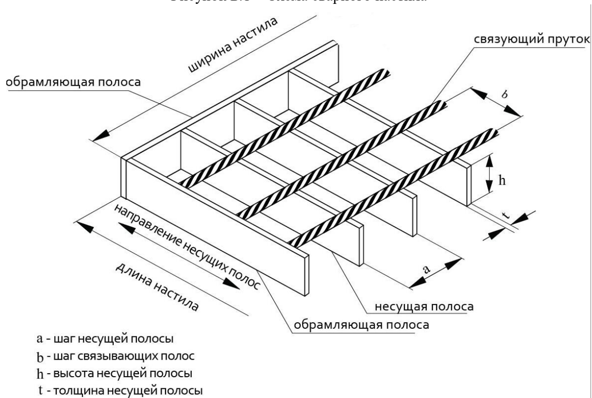
Рисунок Б.1 – Схема сварного настила
